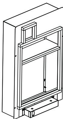
Plénium de Pared (telescopico) RAVWPT15B o RAVWPT15C – 8"-15"D x 23¾"W x 39¾"H
