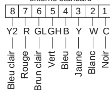
Connecteur de thermostat externe standard
