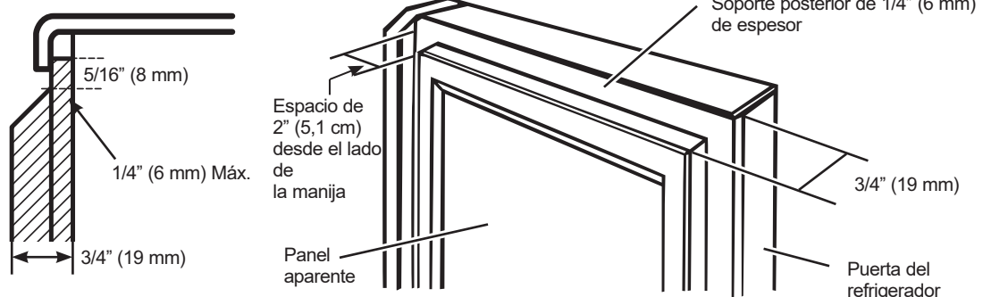
Paneles más gruesos que 1/4" (6 mm)
