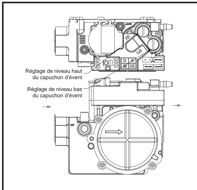
Figure 2. Robinet de gaz à deux niveaux de puissance
