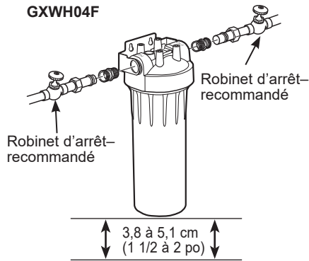
GXWH04F
