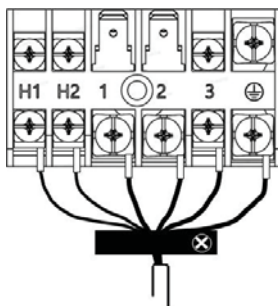
Câblage de commande de l'unité intérieure
