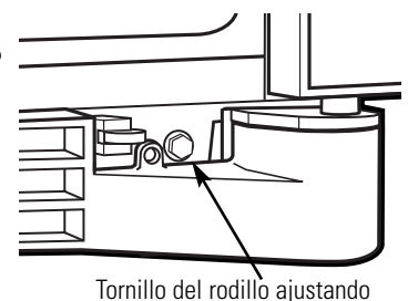
Tornillo del rodillo ajustando
