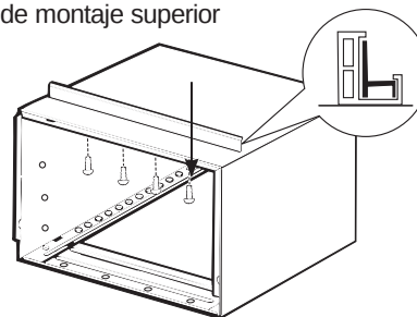
Riel de montaje superior
